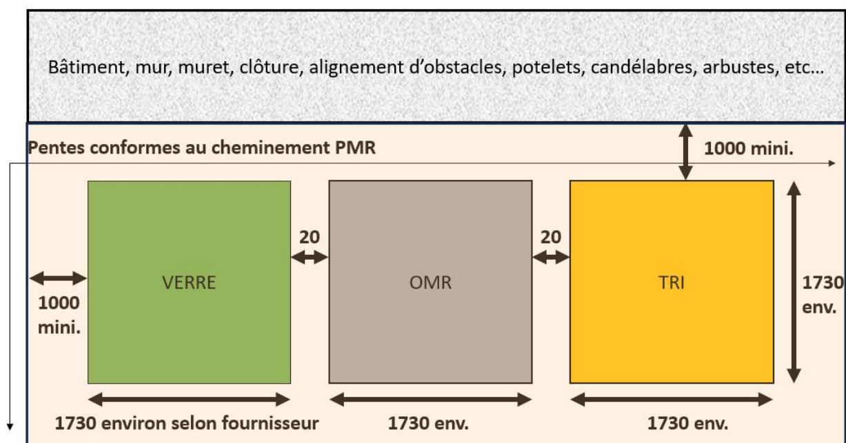
Cas n°1 : Dimensions pour recevoir 3 conteneurs en ligne
